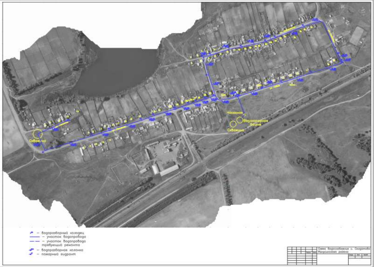
- Схема водоснабжения д. Солдатово – перспективное развитие
