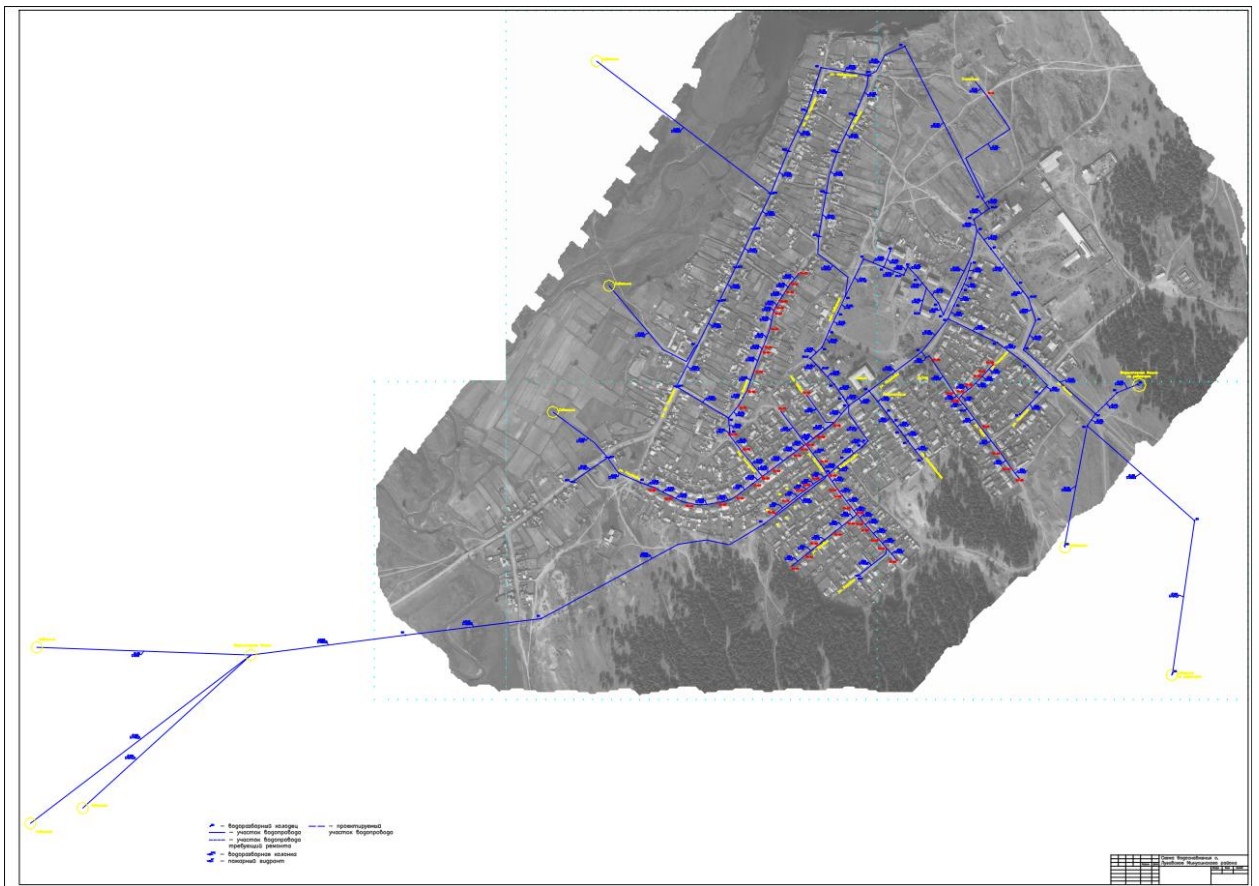
Схема водоснабжения п. Кутужеково
