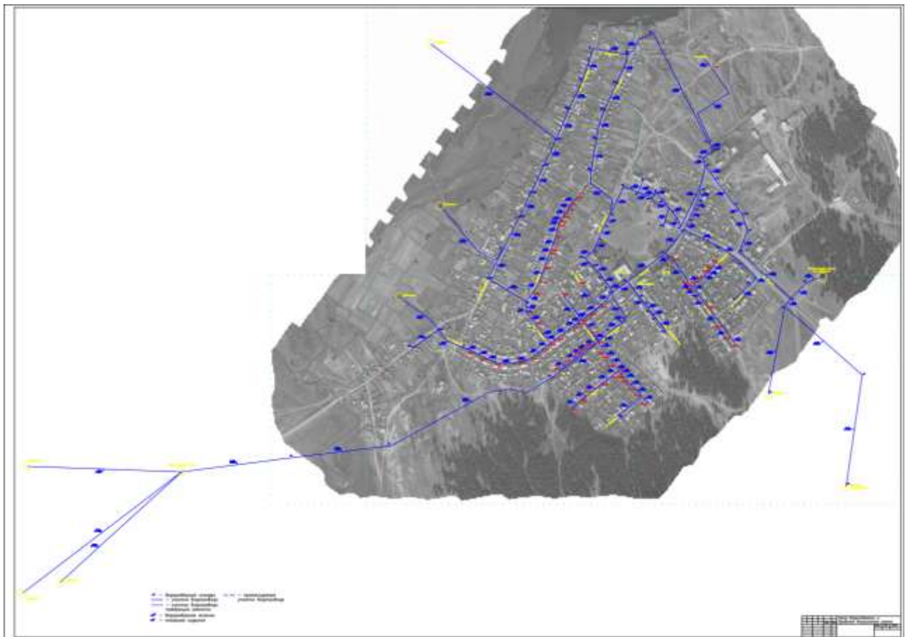
Схема водоснабжения п. Кутужеково
