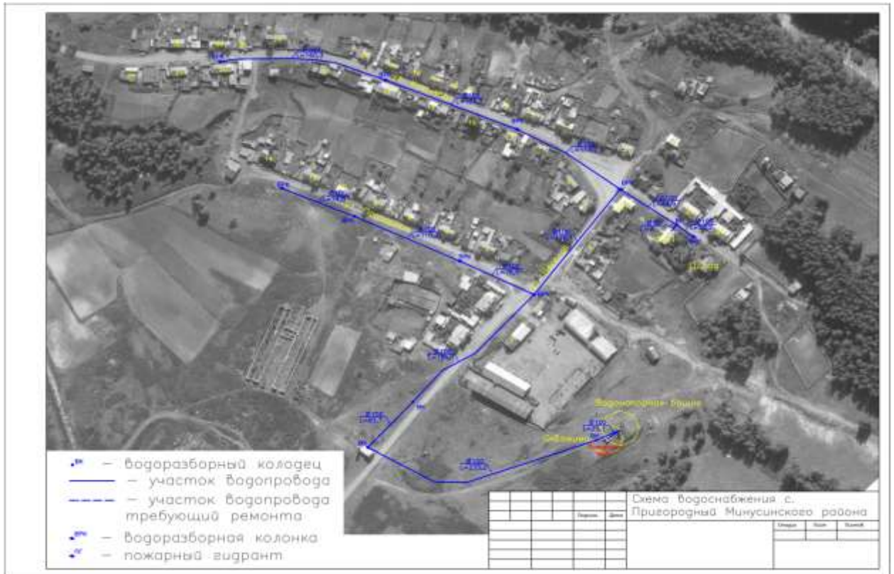
- Схема водоснабжения п. Пригородный
